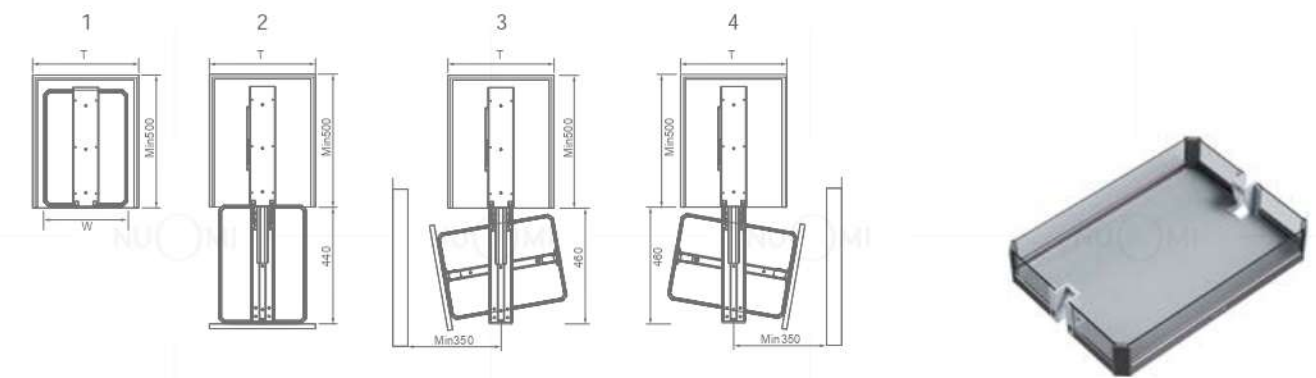
直拉式支架实现状态 /Straight Pull-out Tall Unit : 1、2 180°旋转支架实现状态 /180° Revolving Tall Unit : 1、2、3、4
