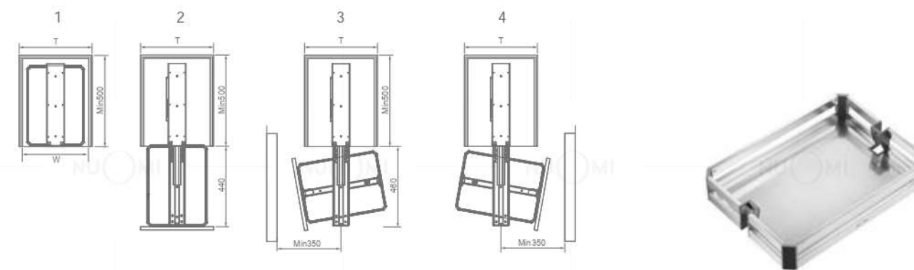
直拉式支架实现状态 /Straight Pull-out Tall Unit : 1、2 180°旋转支架实现状态 /180° Revolving Tall Unit : 1、2、3、4
